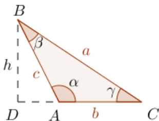
Ilustración 11. Triángulo oblicuángulo
