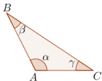
Ilustración 10. Triángulo oblicuángulo
